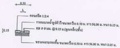
รูปตัดขวางระบบระบายน้ำรูปสี่เหลี่ยม SCALE 1 : 50
