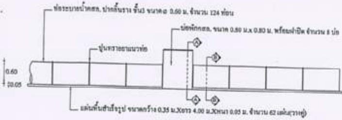
แบบขยายวางท่อคสล.พร้อมบ่อพัก SCALE 1 : 20
