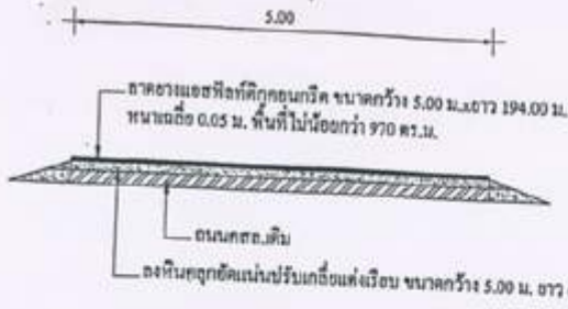
รูปตัด A SCALE 1 : 20
