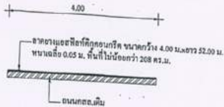
รูปตัด B SCALE 1 : 20
