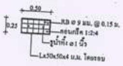
แบบขยายฝ่าปิดบ่อพักคสล. SCALE 1 : 20
