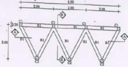
แบบขยายส่วนหน้าหลังคาสัน
