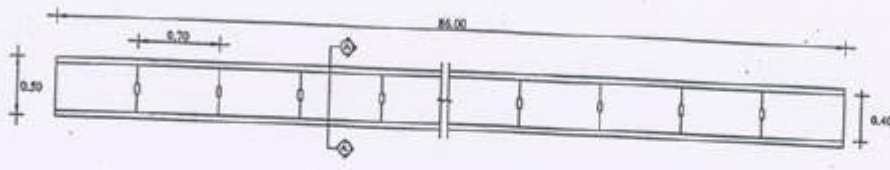
แบบขยายวางระบบน้ำบาดาล SCALE 1 : 20
