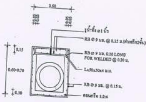
รูปตัด A-A SCALE 1 : 20
