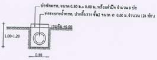
รูปตัด B-B SCALE 1 : 20
