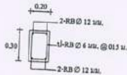
แบบ/จาย B1 SCALE 1:20
