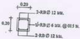
แบบ/จาย C1 SCALE 1:20
