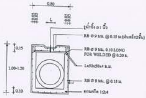
รูปตัด A-A SCALE 1 : 20
