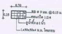
แบบขยายค่าเปิดบ่อพักคสล. SCALE 1 : 20
