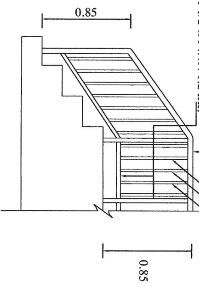
แบบขยายราบบน ไค ยาว 1.60 ม. X สูง 0.85 ม. จำนวน 1 ชุด No Scale
