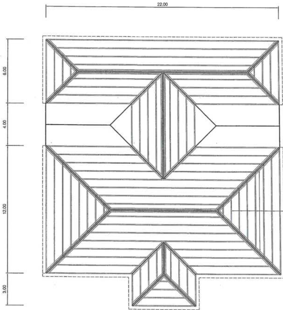
แปลนโครงหลังคา
