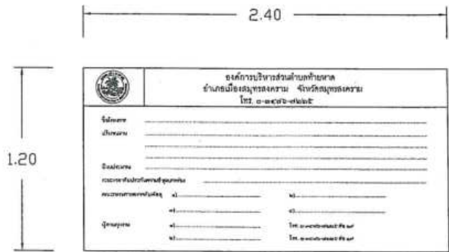
รูปด้านหน้า SCALE 1:20
