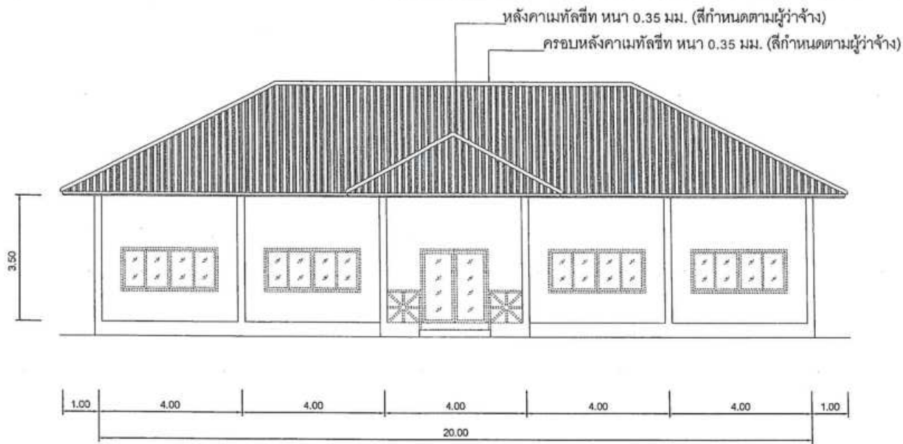
รูปด้าน 1 NO SCALE
