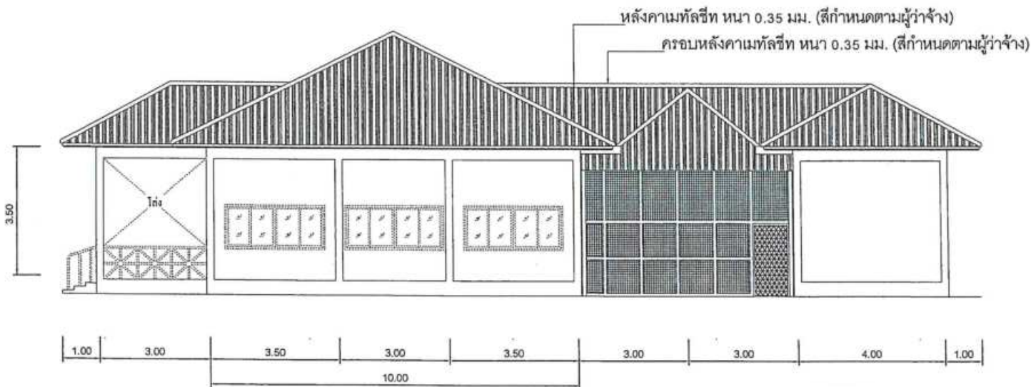
รูปด้าน 2 NO SCALE
